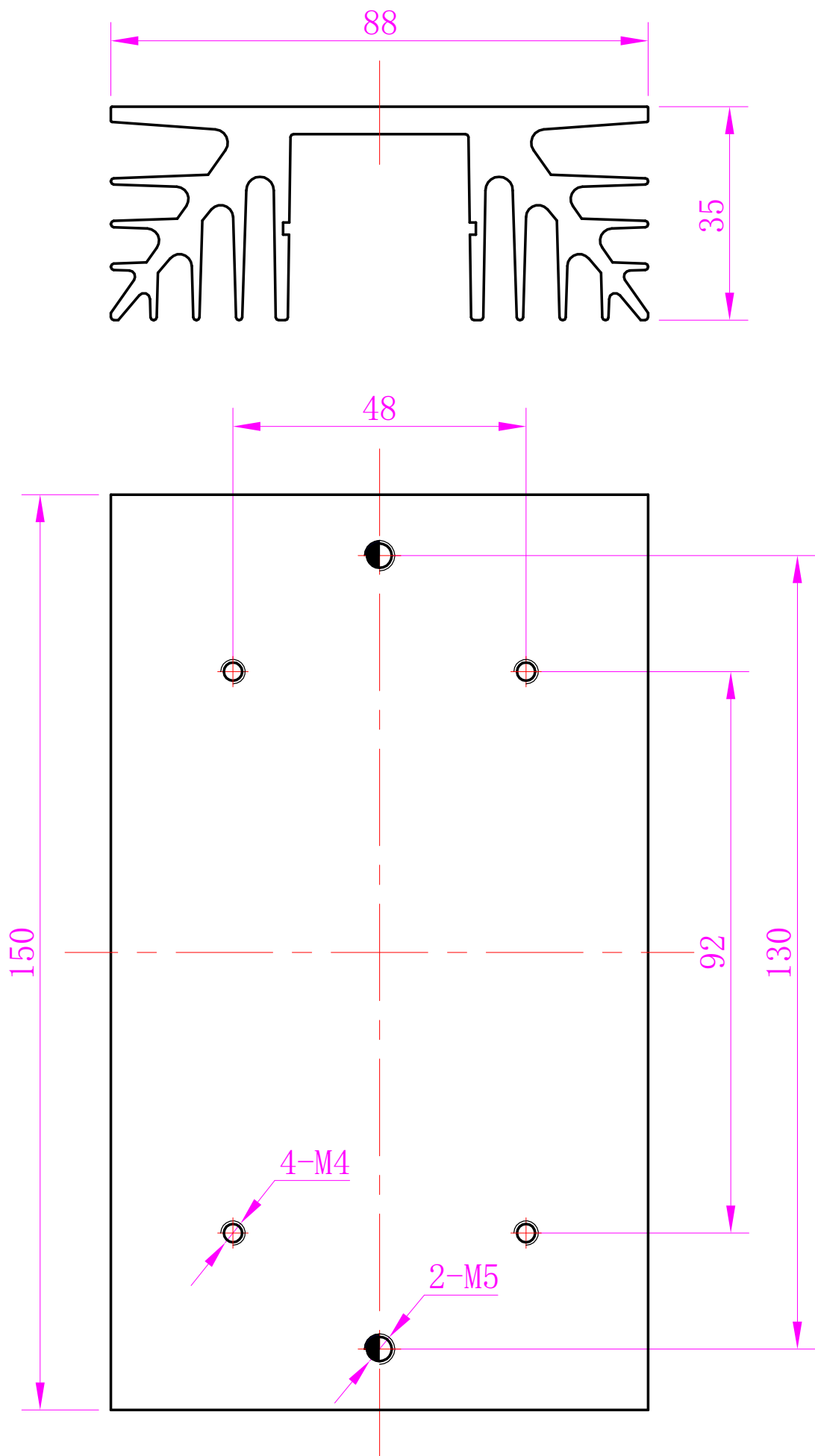
HH-035散热器安装尺寸图
