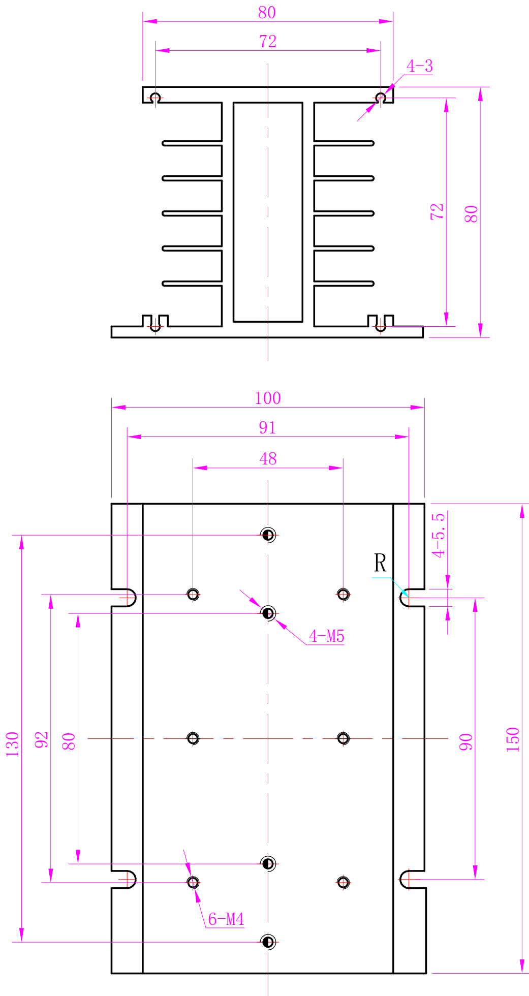
HH-036散热器安装尺寸图
