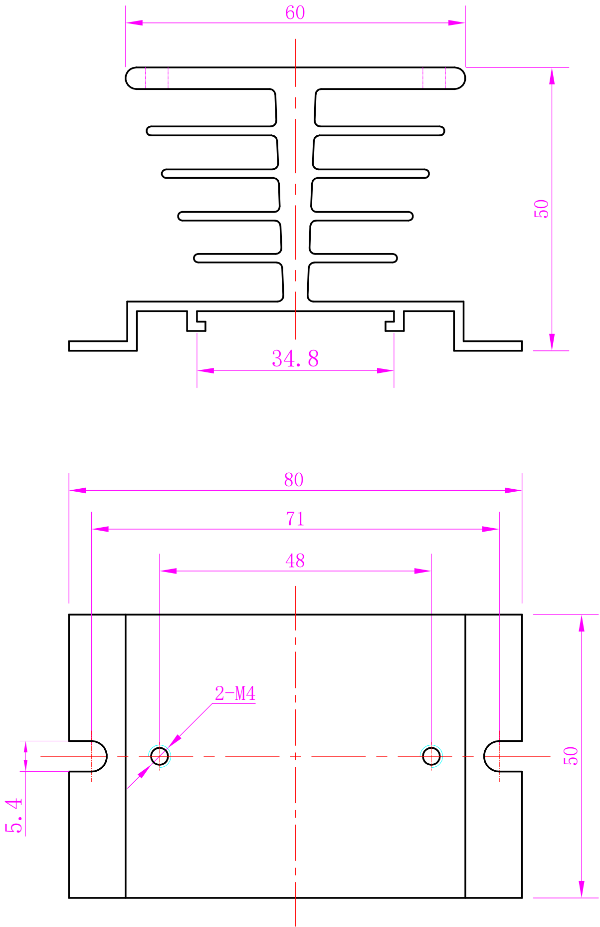
HH-060散热器安装尺寸图
