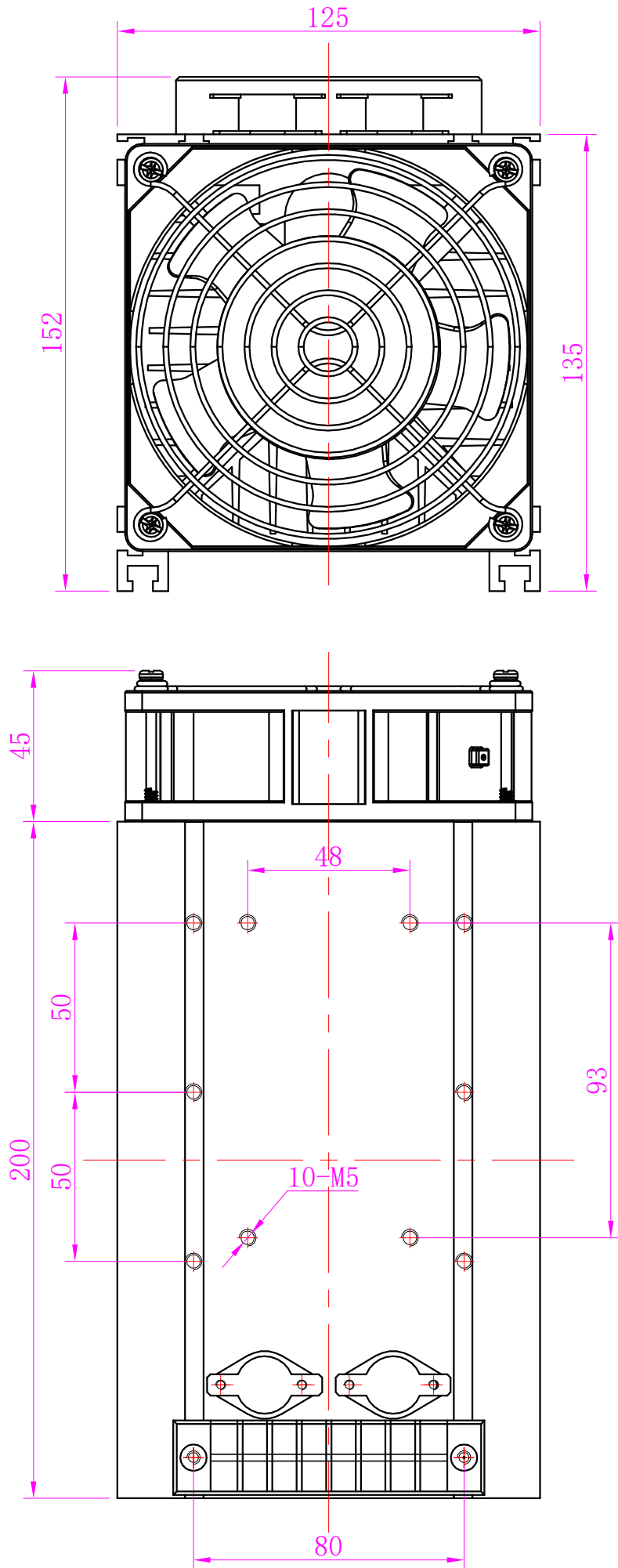
HH-039散热器安装尺寸图
