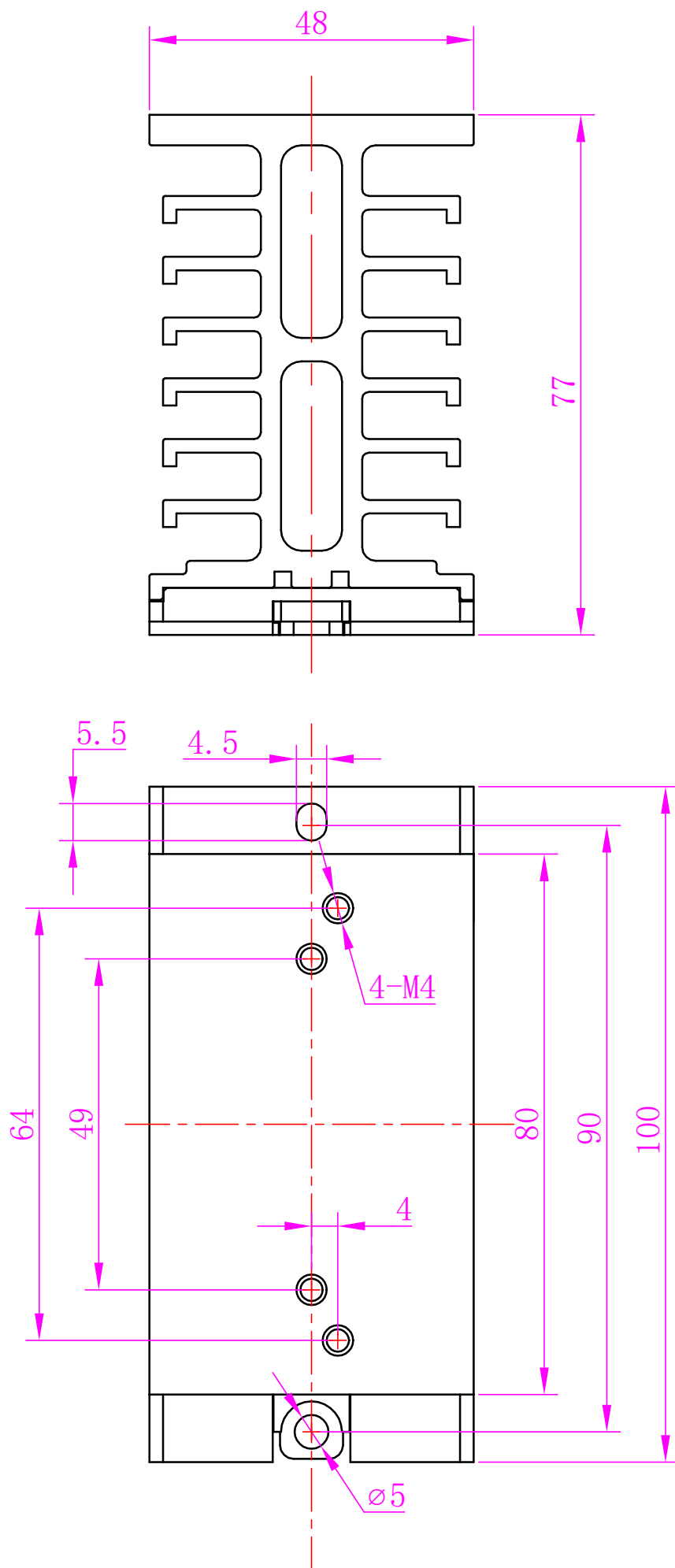
HH-052散热器安装尺寸图
